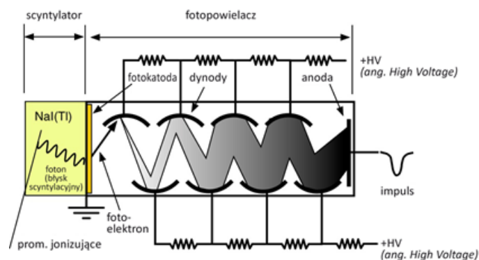
Rys.2 Budowa detektora scyntylacyjnego
